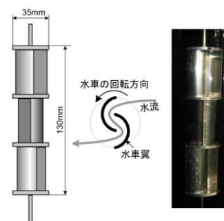
波力発電システムの実験装置
