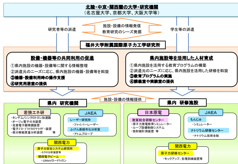
嶺南地域原子力関連施設の共同利用スキーム(案)
