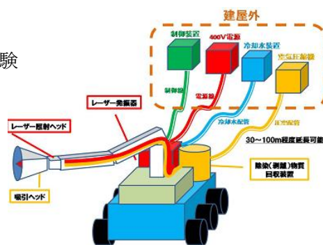
レーザー除染装置 (イメージ図)
