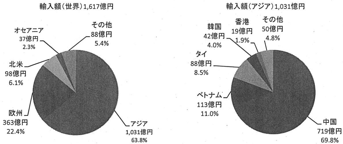
(図2) 県内企業の地域(国)別輸入額(2015年)
