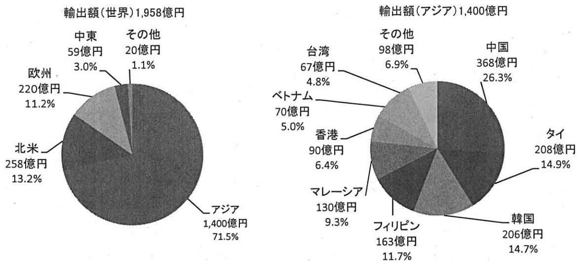
(図1) 県内企業の地域(国)別輸出額(2015年)
