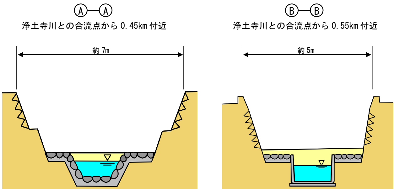
図 5.17 横断面図
