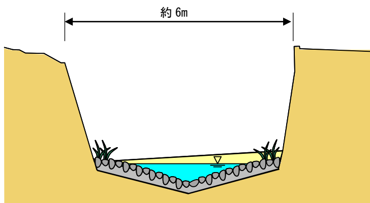
図 5.18 横断面図
