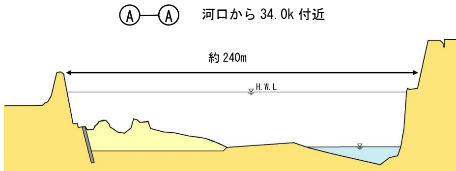
図 5.4 横断面図
