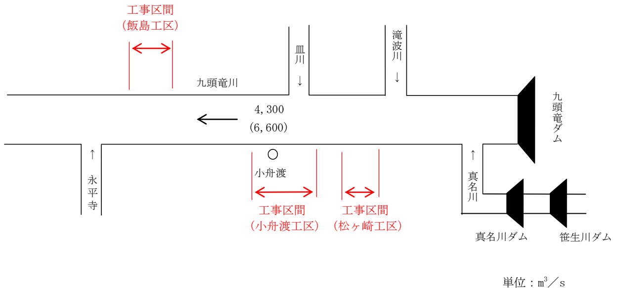
図 5.2 計画流量配分図
