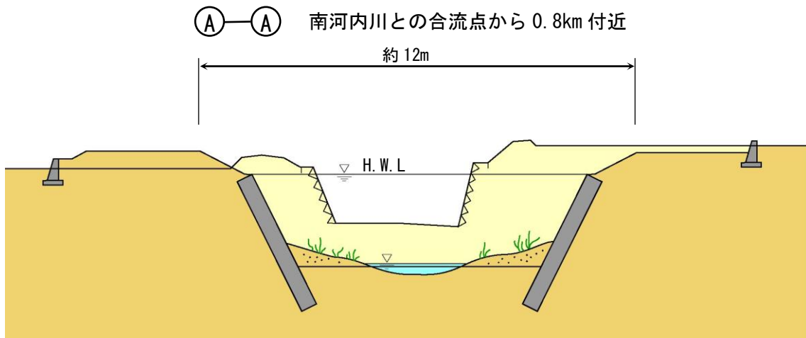
図 5.14 横断面図
