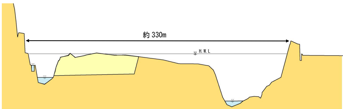
図 5.6 横断面図
