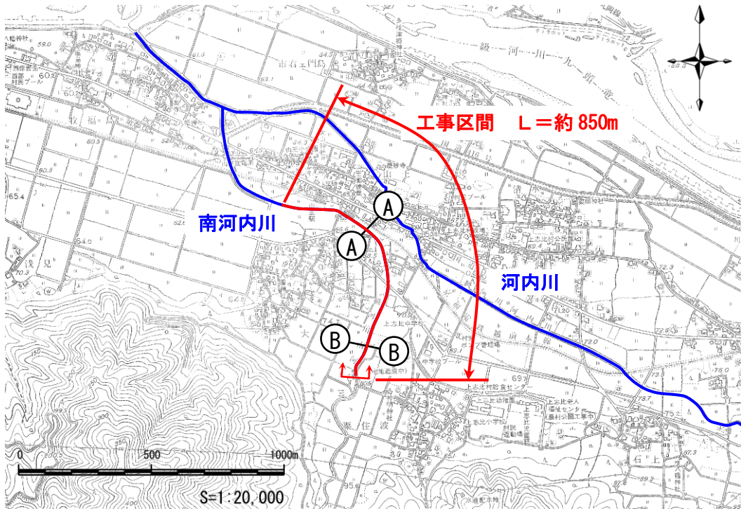
図 5.10 平面図
