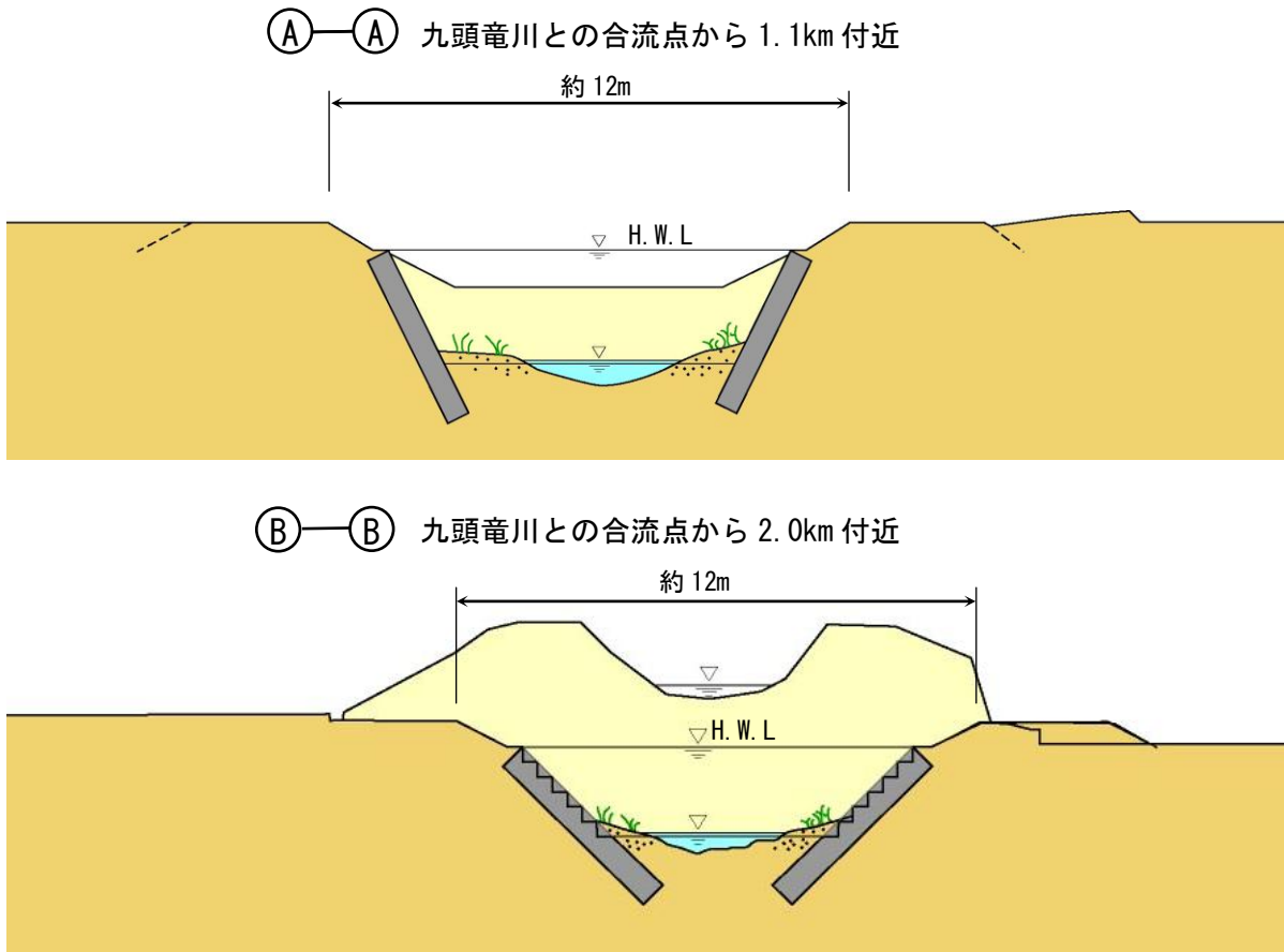
図 5.11 横断面
