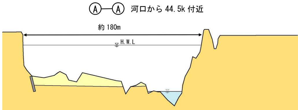
図 5.8 横断面図
