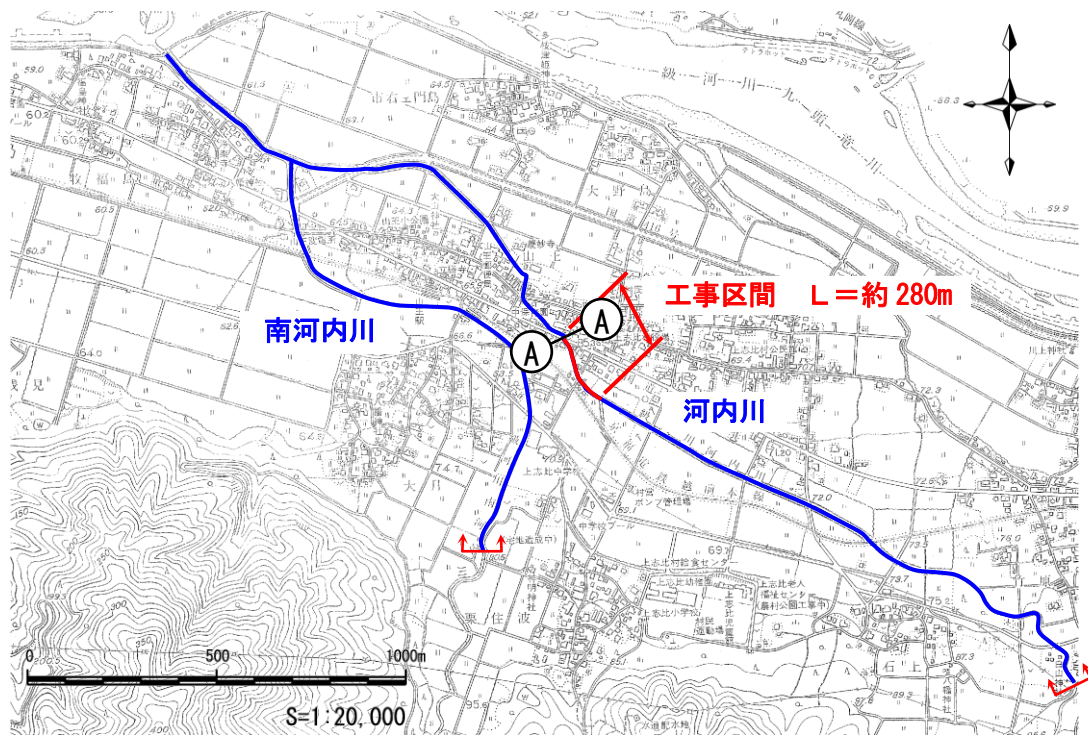
図 5.13 平面図
