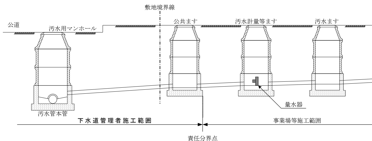
量水器及び試料採取口設置例標準横断面図
