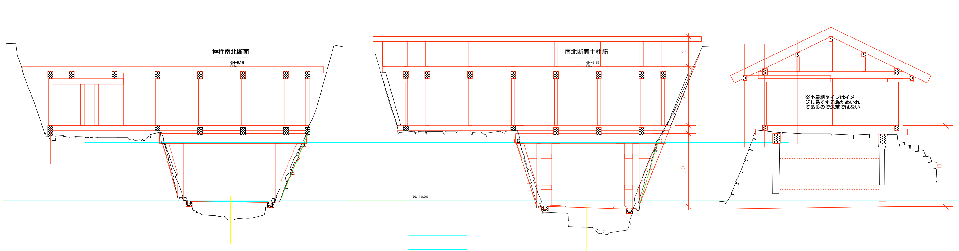
図4の平面図の場合の柱梁位置想定図
