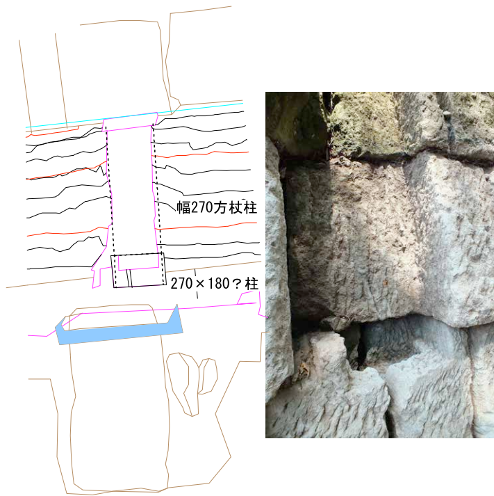
写真 1 支柱筋の北石垣柱痕跡
