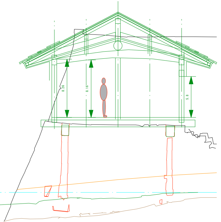
桔木型（丸岡城型）
