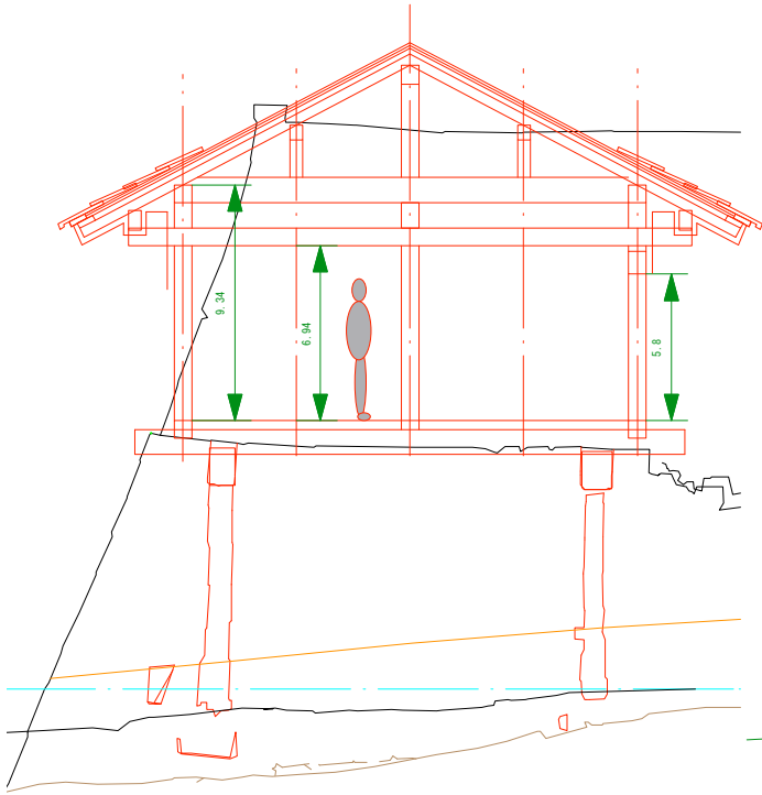
梁跳ね出し型（福井城天守型） 梁が低い
