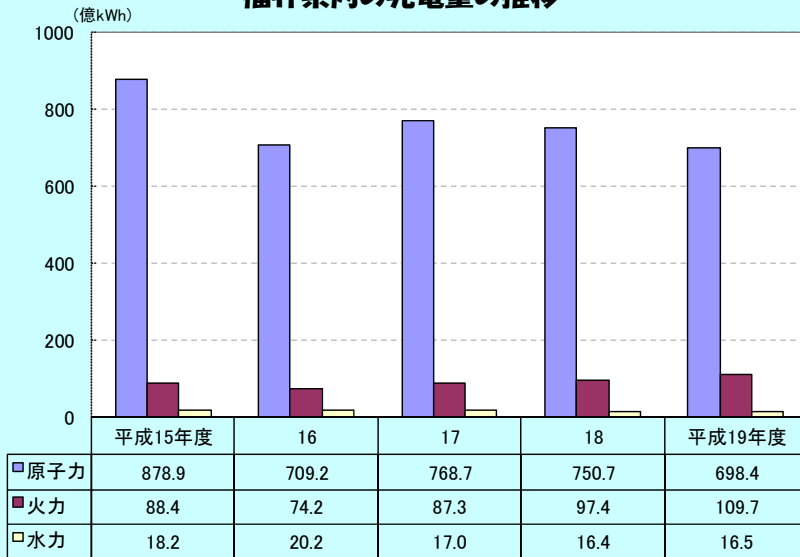
福井県内の発電量の推移
