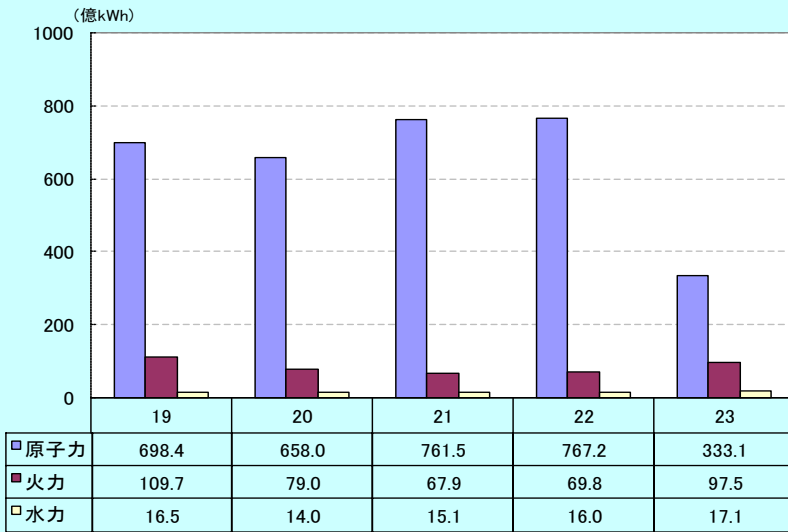
福井県内の発電量の推移
