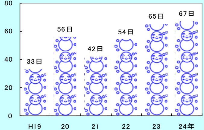
年間雪日数(福井市)
