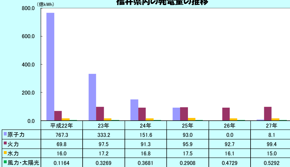
福井県内の発電量の推移
