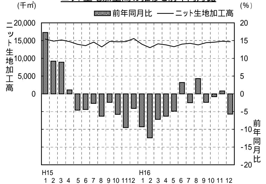
ニット生地加工高の推移と前年同月比
