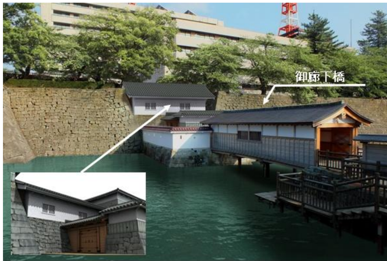
山里口御門復元予想図
