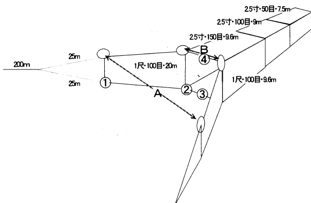
図1 駆除網模式図
