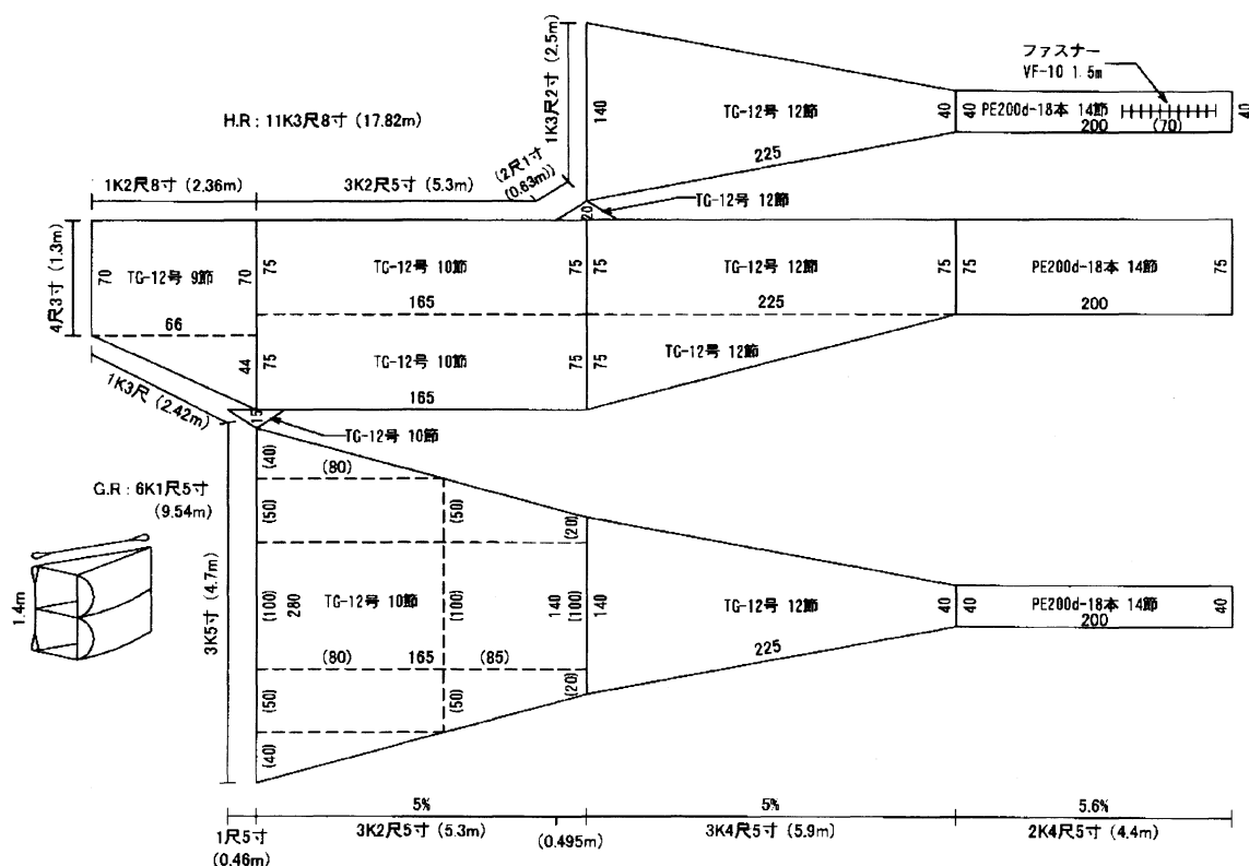
図 8 作製した船びき網の展開図と拡網装置の概略図
