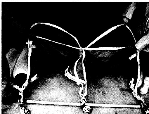
図 9 作製した拡網装置
