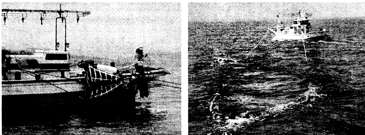
図 11 漁船による曳網試験の状況
