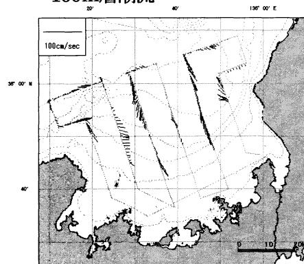
100m層潮流
