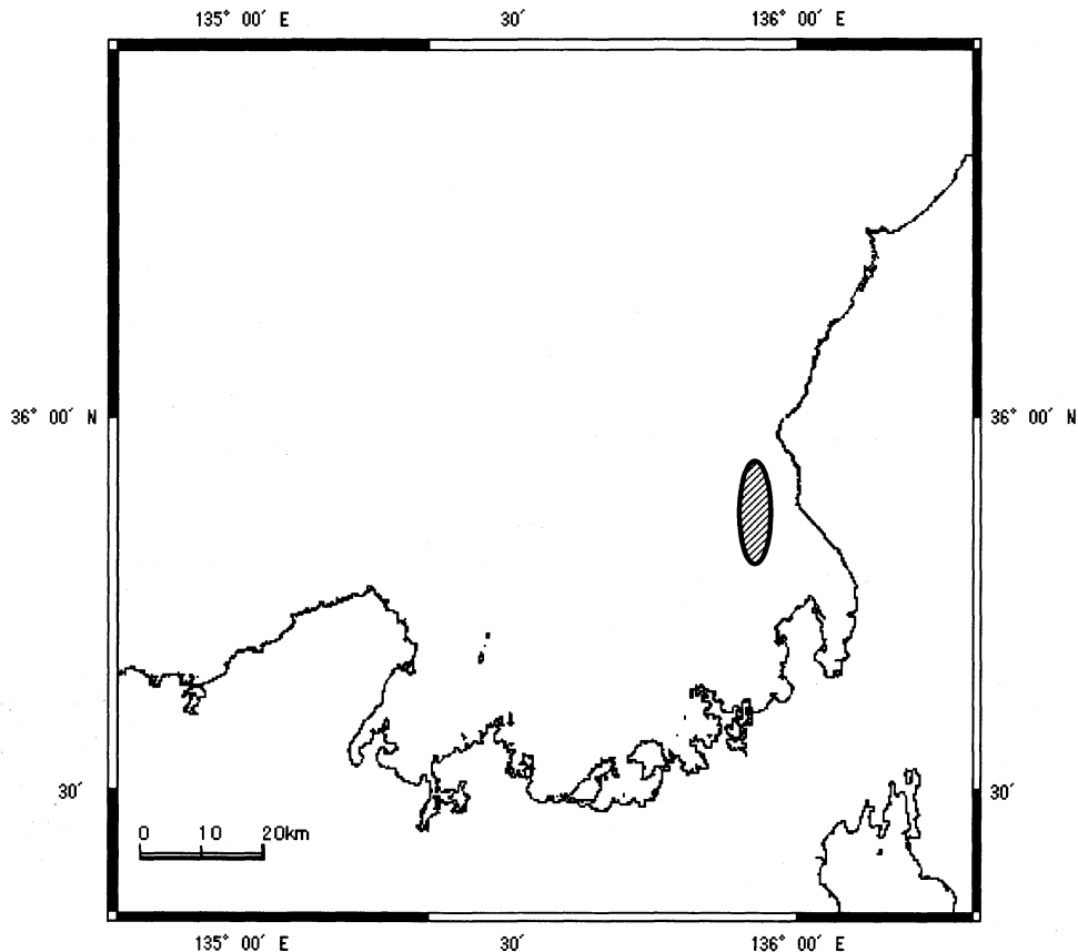
図 1. 調査位置
