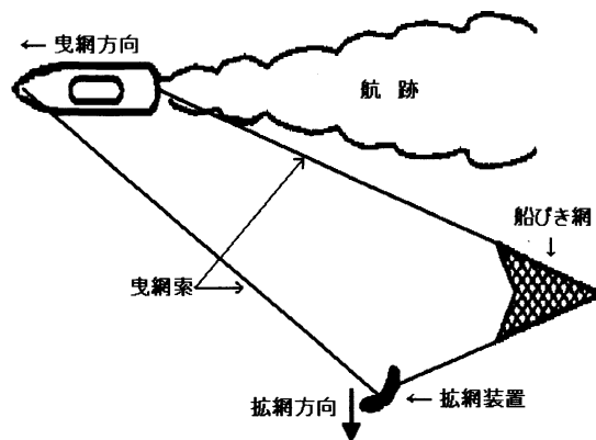
図 10 1 隻での曳網概要図
