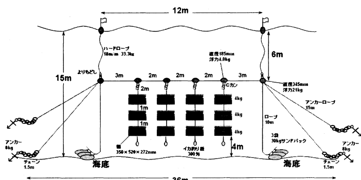
図3 簡易越夏施設図
