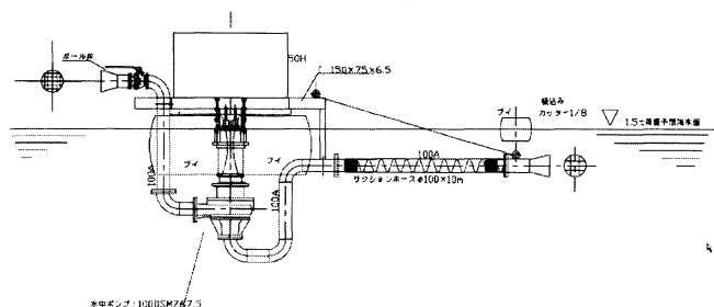
図 2 ポンプ式大型クラゲ駆除装置
