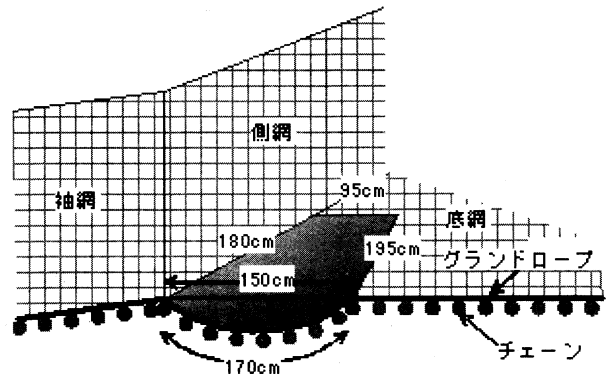
図2 カイト模式図
