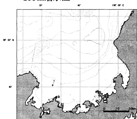
150m層水温
