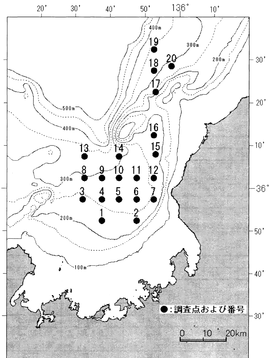
図4 調査定点
