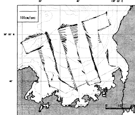
50m層潮流
