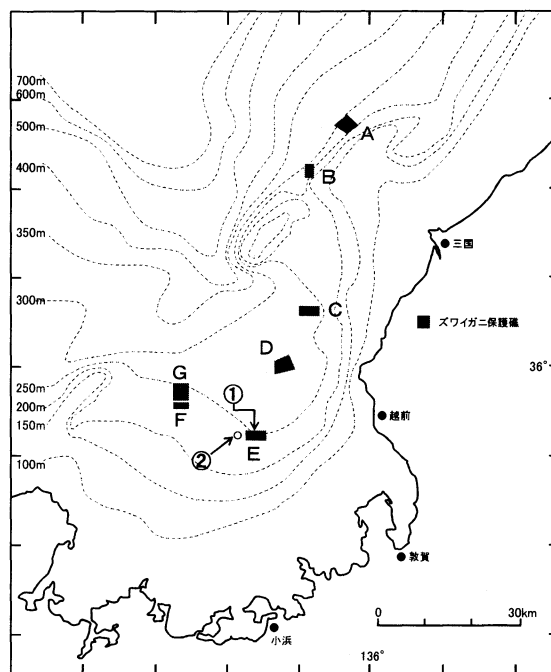
図1 調査海域図
