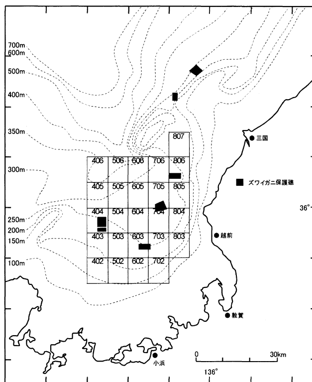
図 1 調査海域図
