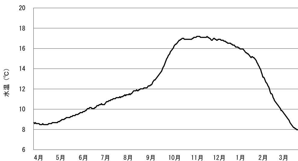
図2 新飼育棟における使用地下水の水温（令和3年4月～令和4年3月）
