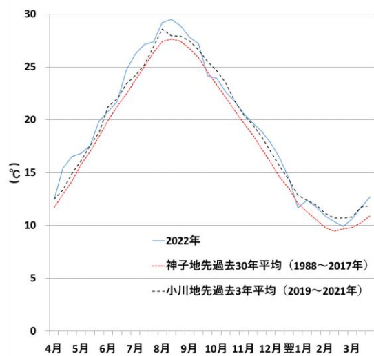
図4 小川地先における表面水温の推移
