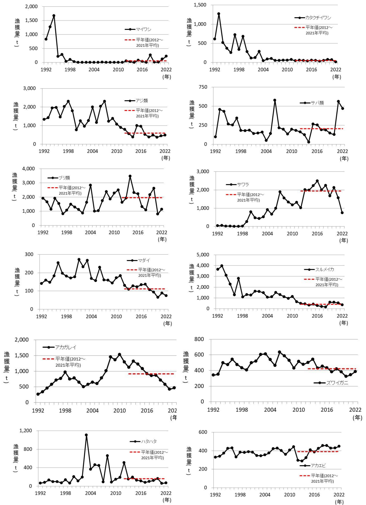
図 6 県内主要魚種の経年変化
