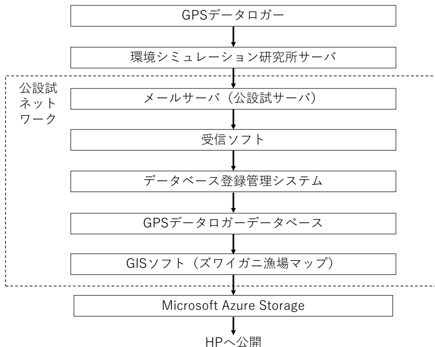
図2 稚ガニの入網情報提供のスキーム
