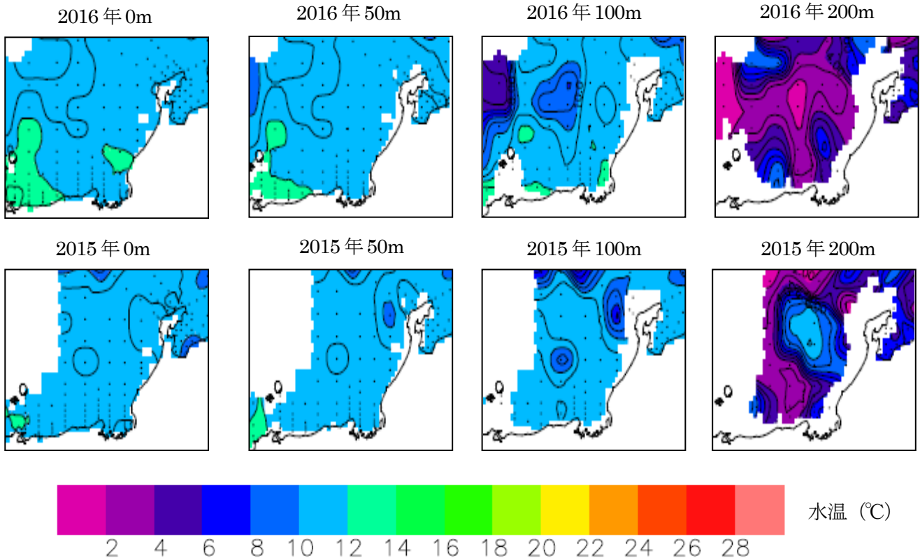
図3. 福井県およびその周辺海域の水温分布図 (日本海区水産研究所の日本海漁場海況速報より抜粋)
