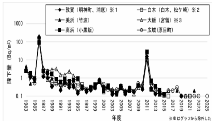
図2-3 セシウム-137の年間降下量の推移
