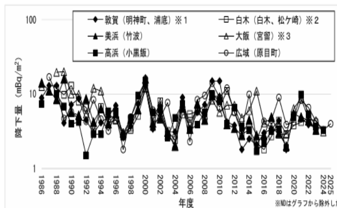
図2-5 プルトニウム-239の年間降下量の推移
