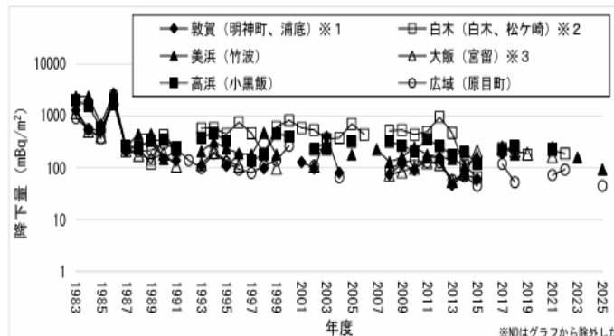
図2-4 ストロンチウム-90の年間降下量の推移
