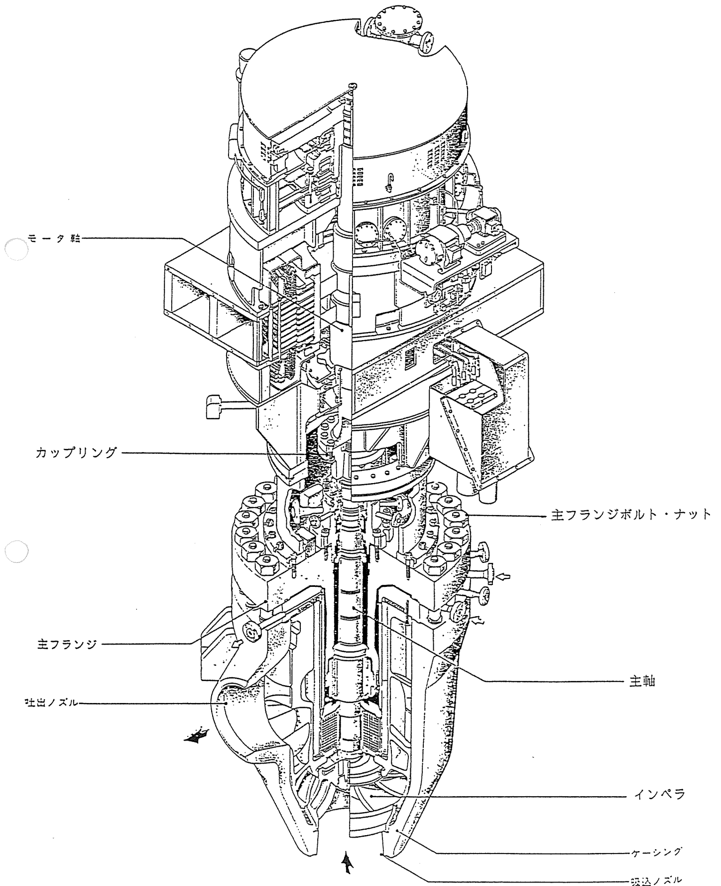
図 - 1 1 次冷却材ポンプ構造図
