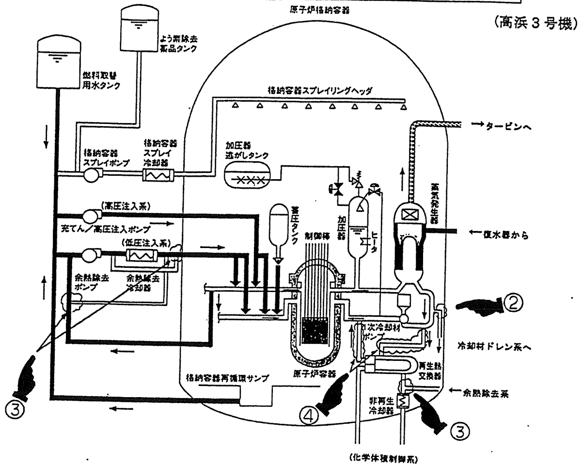
図-3 敦賀2号機 一次冷却水漏えい事故反映 検査充実概要図
