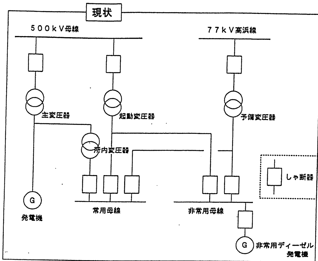
図-2 発電機負荷開閉装置設置工事図
