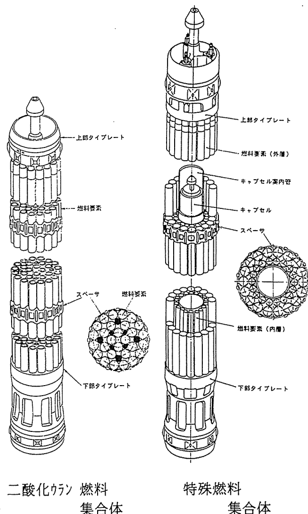
構造図
