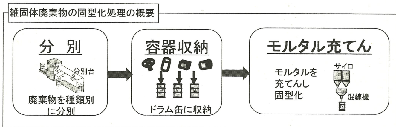
第3図 固体廃棄物処理系統図(1号及び2号炉の例)
