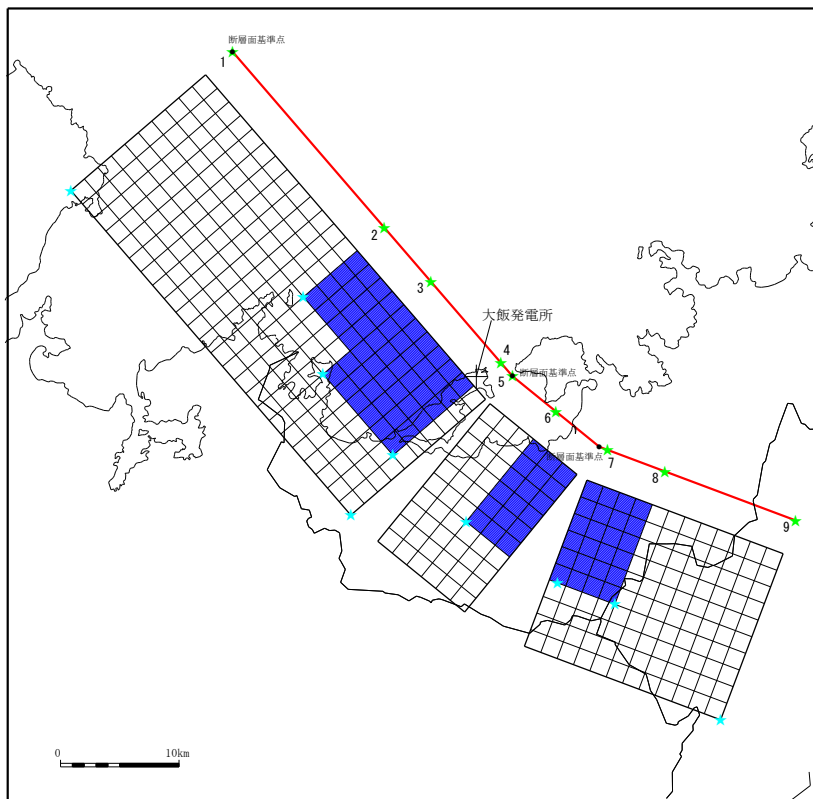
断層配置図
