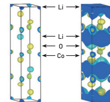
LiCoO 2 電池正極のリチウム密度の変化とLiの拡散経路
