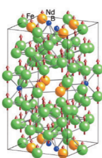
ネオジウム磁石の結晶構造 [出典: 日本中性子科学会 「N氏の新たな冒険」より転載]
