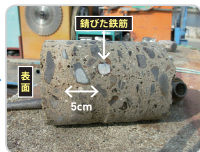
コア抜きしたコンクリート表面から1cm間隔で試料を採取
