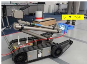
レーザー除染システムを搭載する小型ロボットのイメージ (例：PackBot)
