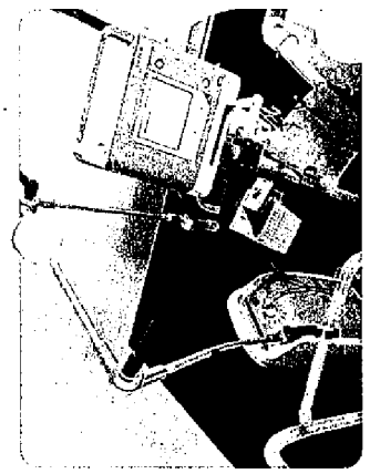
人工呼吸器(右)、肺や気管にたまる痰を排除する排痰装置「エアスクリーン」(左)
