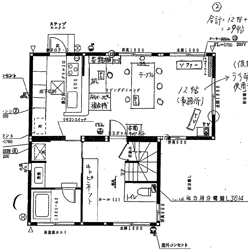
1階平面図
