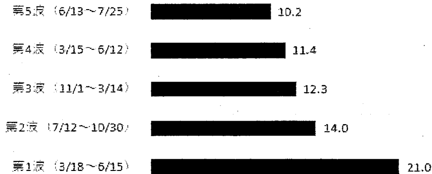
陽性者数と入院者数推移
