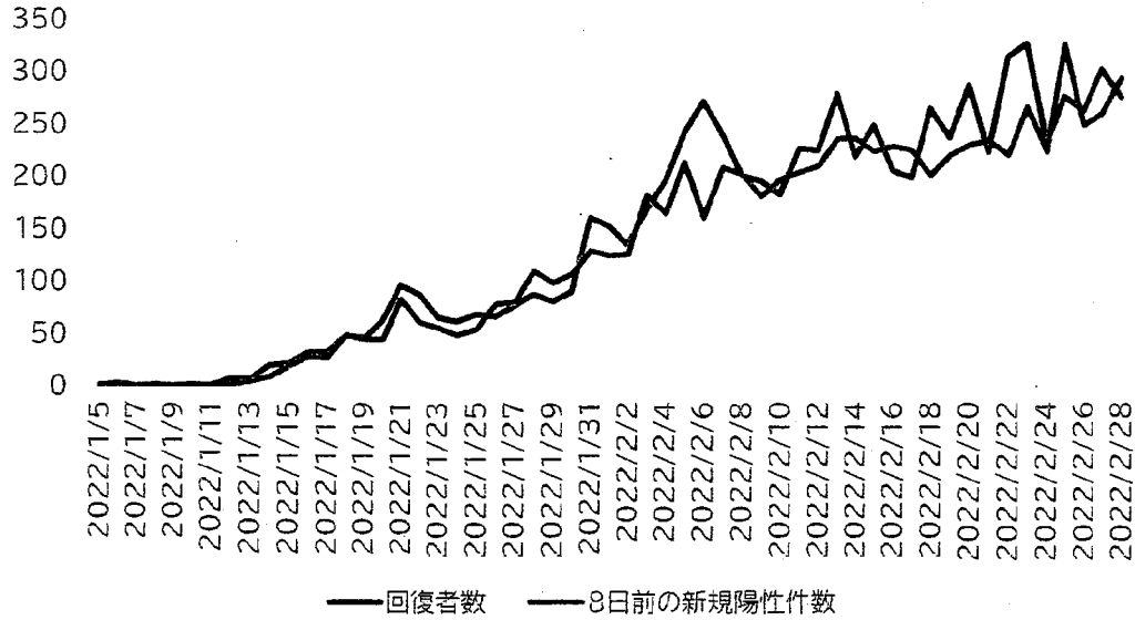
回復者数と8日前の新規陽性者数
