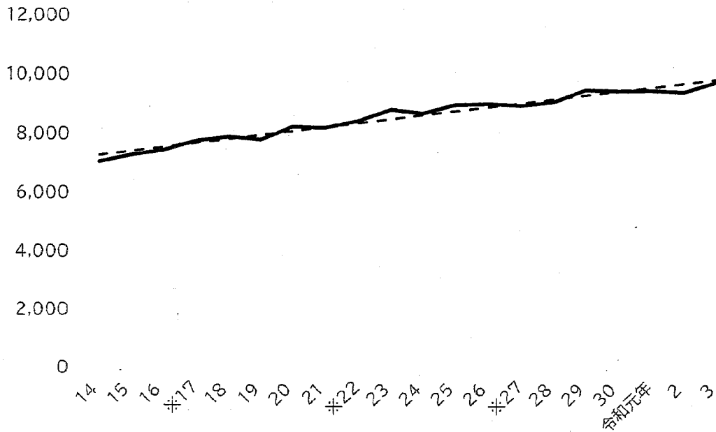
福井県の死亡数推移
