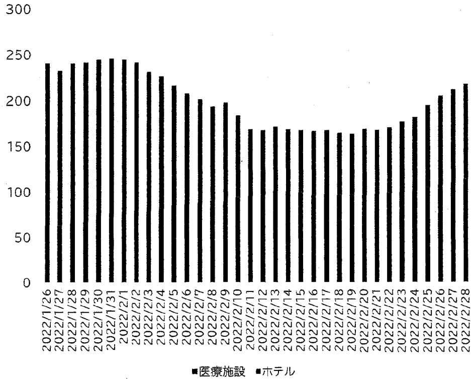
福井県入院患者数推移
