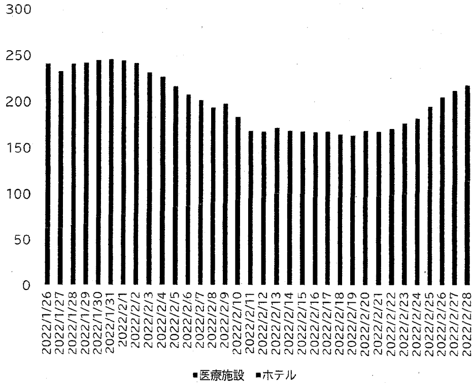
福井県入院患者数推移
