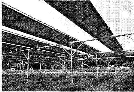
福島県農民連のソーラーシェアリング(営農型太陽光発電・写真、県内にある市民・地域共同発電所は12の基で全国のなかでも多い)「原発の電気は使いたくない」との思い、「2040年頃には県内エネルギー需要の100%相当量を再生可能エネルギーで」と目標掲げる県の姿勢がある(7面)
