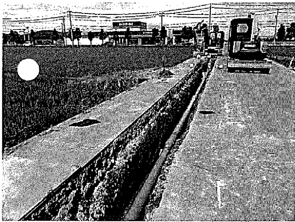
末端パイプライン施工状況
