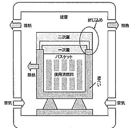
[乾式]金属キヤスク貯蔵方式
