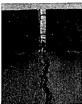
湖岸堤防と管理道路の亀裂
