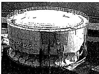
津波の力で凹んだタンク
