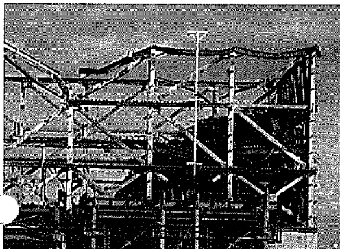
福島第一原発1号機は水素爆発事故当時のまま
