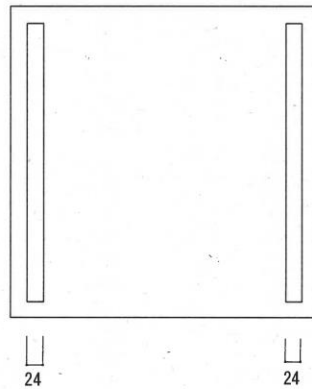
天端板
