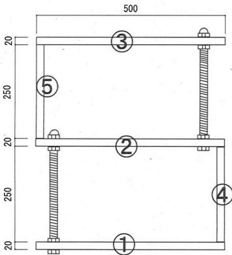
正面図
