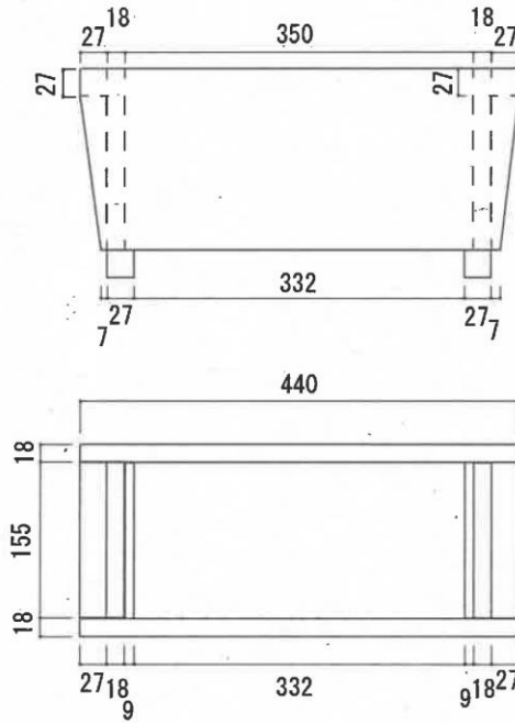
平面図
