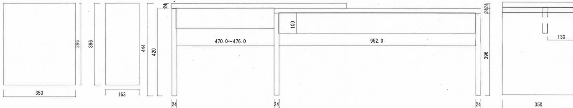
平面図
