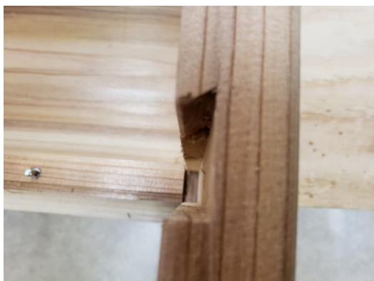
溝加工 (例)
