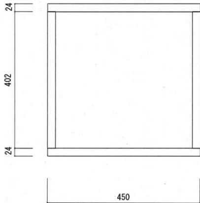
平面
