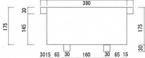
正面図
