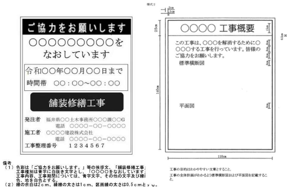
図1-1-2 標示板の例
