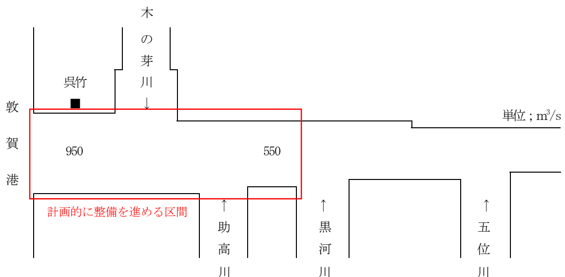
図 3.4.1 筈の川水系の整備目標流量図
