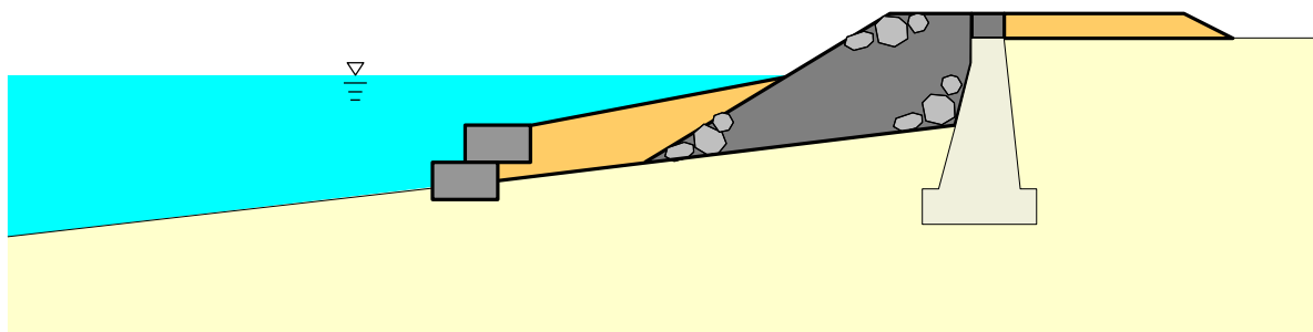
図 4.1.5 湖岸堤嵩上げの横断面図（イメージ）
