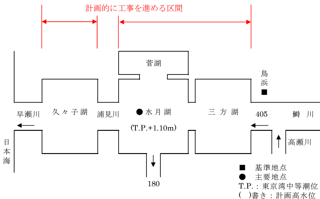
図 4.1.2 計画流量配分図 (単位：m³/s)
