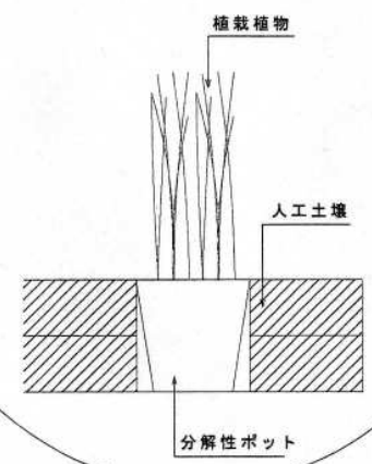
植栽箇所断面図
