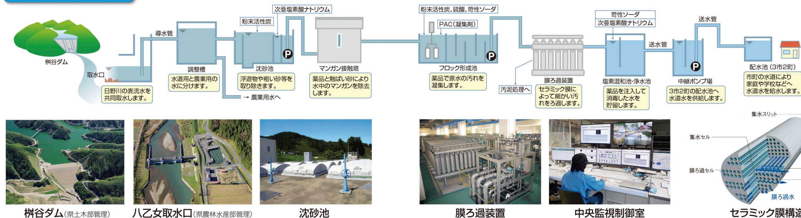
浄水場全景
