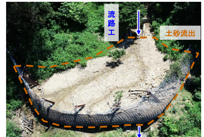
【土砂流出防備保安林(福井市蒲生町)】 土砂流出による被害を防ぐため治山ダムを復旧 (大量の土砂を透水型治山ダムにより堰き止め、 民家や国道等の甚大な被害を防止)
