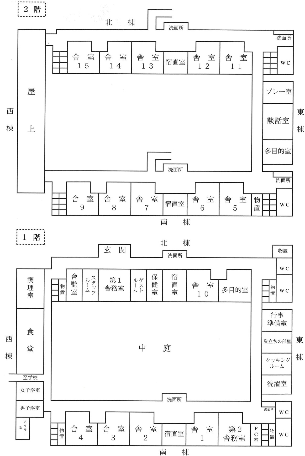
17 寄宿舎平面図
