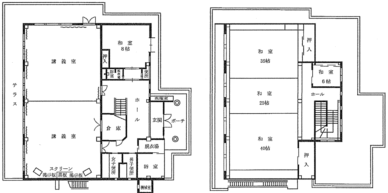
1 階平面図
