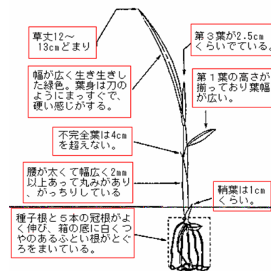
目標とする稚苗の姿 (星川氏原図から作成)
