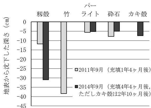
第9図 資材の耐久性
