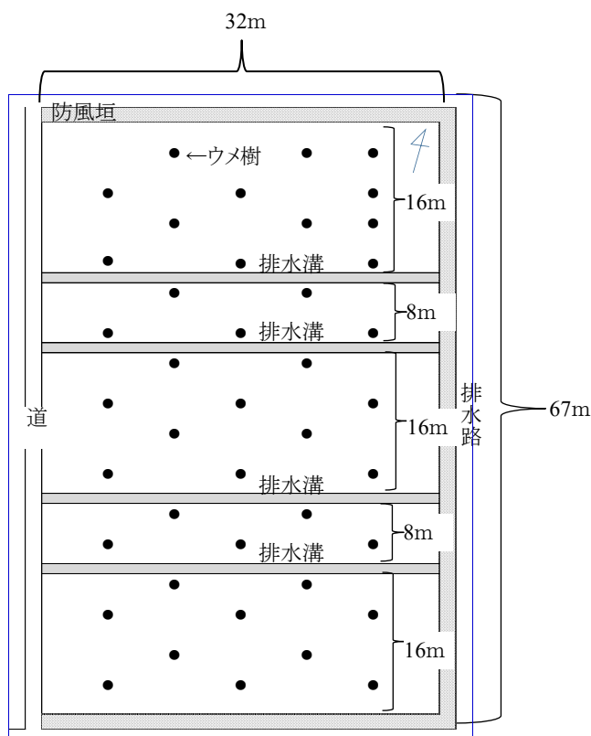
第 1 図 水田転換改良園の模式図
