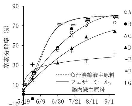
第 1 図 窒素分解率の推移（2014）
