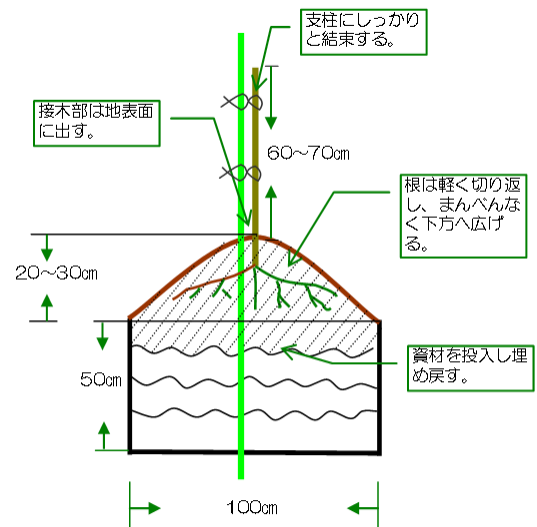
図5 苗木の植付け方法
