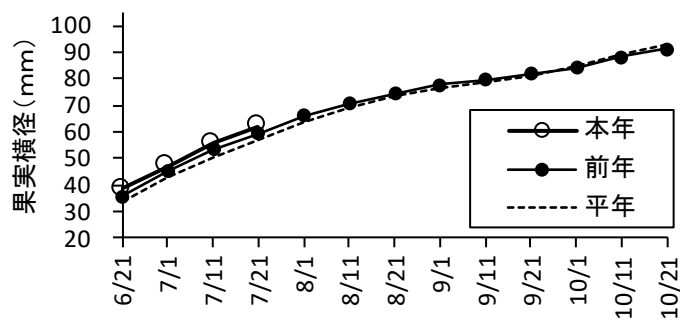
図6 「平核無」の果実肥大
