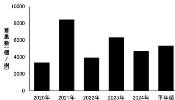
図2 「紅サシ」の総着果数
