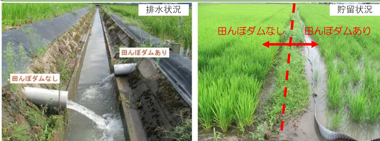
写真 「田んぼダム」のありなしによる排水状況の違いと貯留状況の違い
