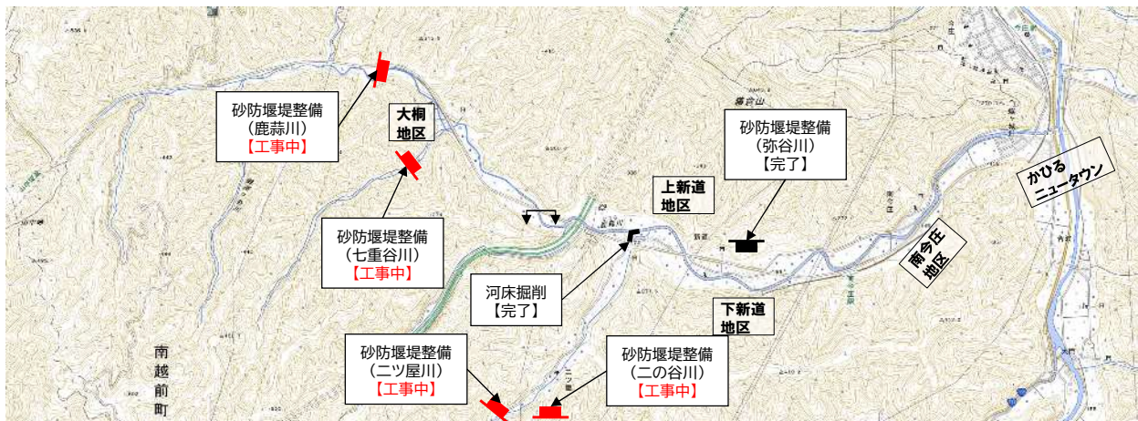
鹿蒜川砂防堰堤 [大桐地区]
