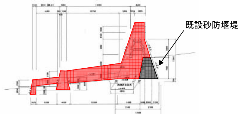
既設砂防堰堤：不透過型ダム
