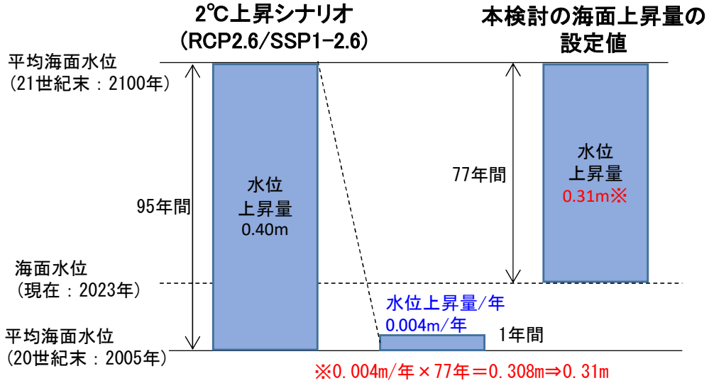
海面上昇量の模式図
